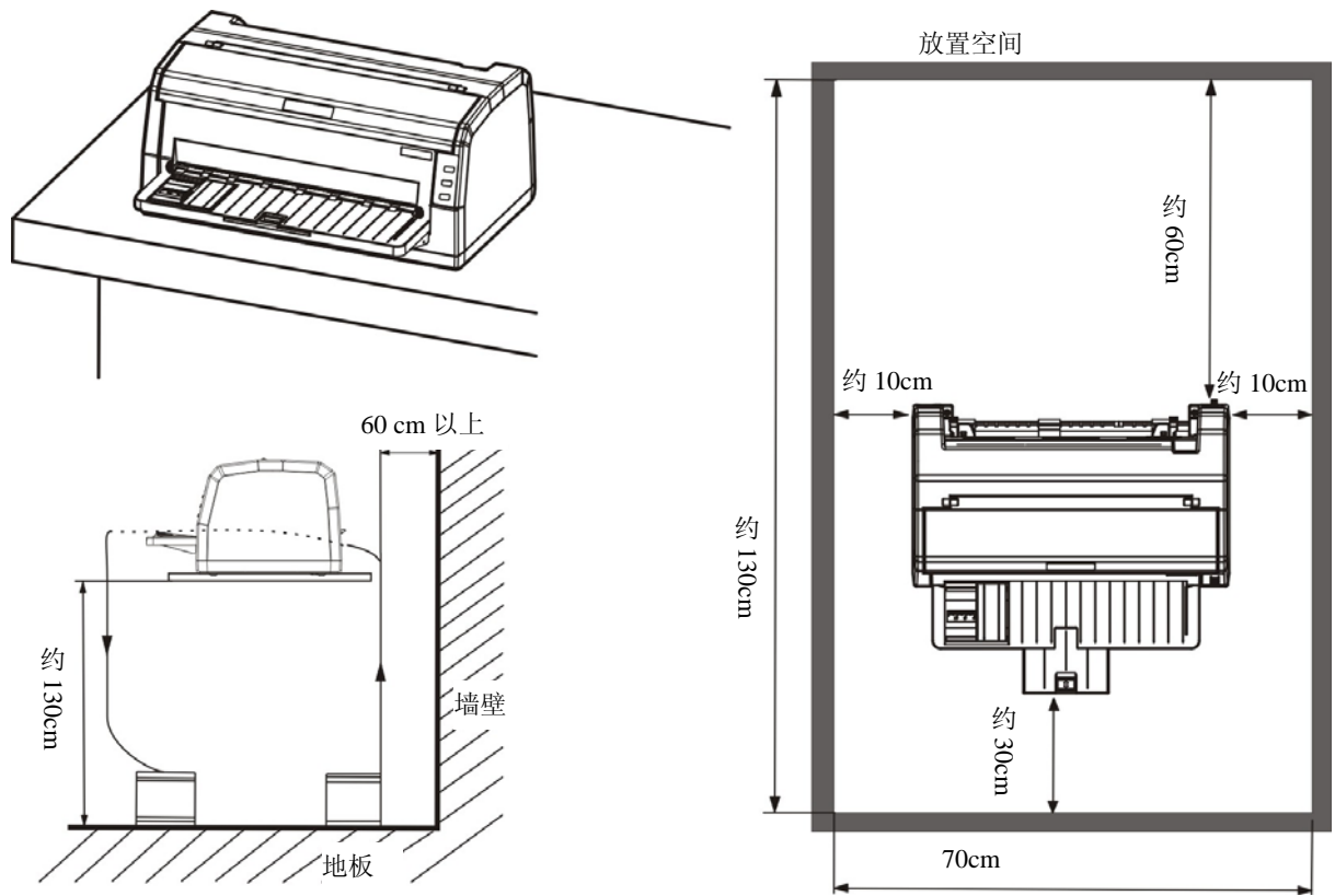
图 2-4 打印机放置
